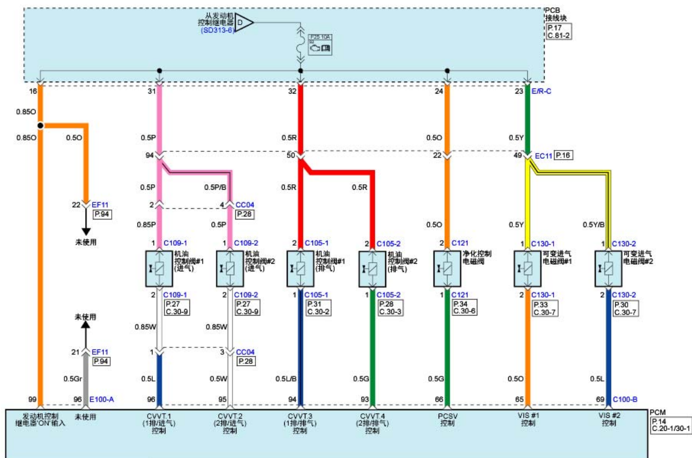
发动机控制系统(G6DH : LAMBDA II 3.3L GDI)(7)
